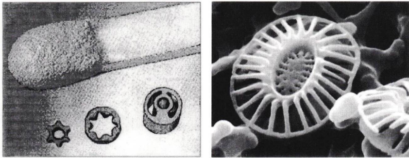
Abb. 4. In der heutigen Mikrotechnik ist man stolz auf Zahnradchen von \frac{1}{2} mm Durchmesser, bei einer Formtoleranz von \frac{3}{1000} mm. Die Natur im Vergleich: Ein ganzer Coccolith misst nur \frac{4}{1000} mm im Durchmesser, die einzelnen Speichen sogar nur \frac{8}{100\,000} mm (80 nm) – bei einer Präzision, von der Techniker nur träumen können. 12'500x.
