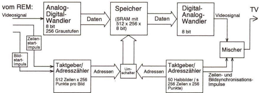
Abb. 9: Blockschema des Bildspeichers
