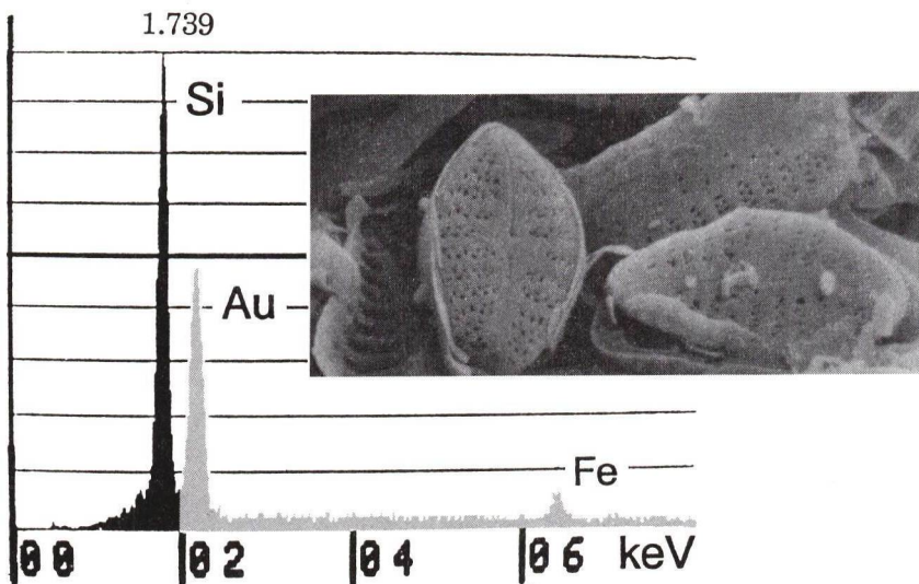
Abb. 12: Analyse fossiler Kieselalgen (ca. 8. Millionen Jahre alt; Vergr. 2'000 X): Das Skelett aus Kieselsäure ( \text{SiO}_2 ) zeigt sich deutlich im scharfen Silizium-peak (Si) bei 1.739 keV; der Gold-peak (Au) rührt von der Präparatbehandlung (Goldbedampfung) her; auch Spuren von Eisen (Fe) lassen sich nachweisen.
