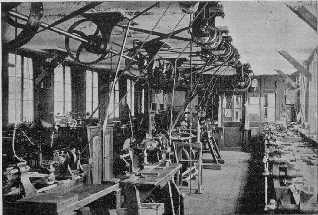
Partie aus einem Atelier der Reißzeugfabrik Gysi & Cie. in Aarau. Nach Photographie Gysi & Cie.
