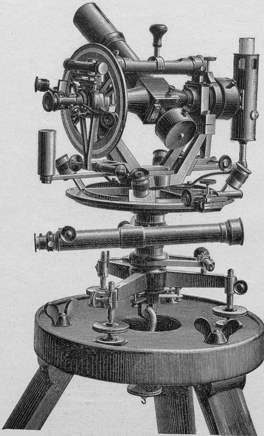
Universaltheodolit.
